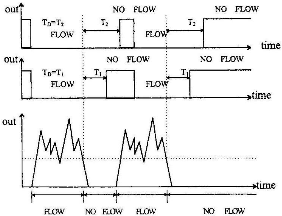
图4、工作曲线
