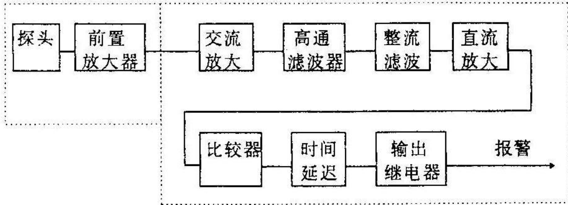
图 3、 流程框图
